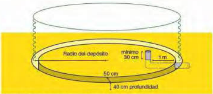
Figura 1: Perfil de la regata (zanja) y tubos de salida de agua.
