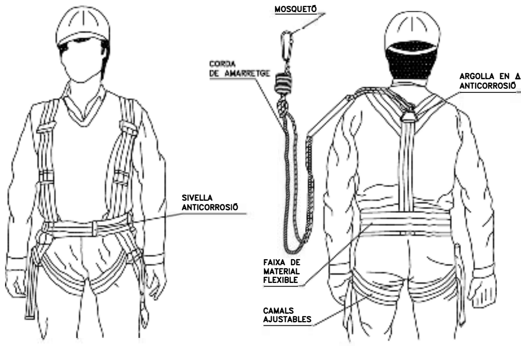
ARNES DE SUBJECCI3 DAVANT CAIGUDES
