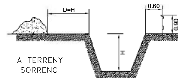
PROTECCI3 EN RASES
