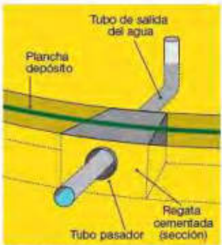
Fig. 3: Detalle del tubo pasante.
