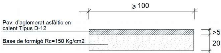
Detall reposició asfalt
