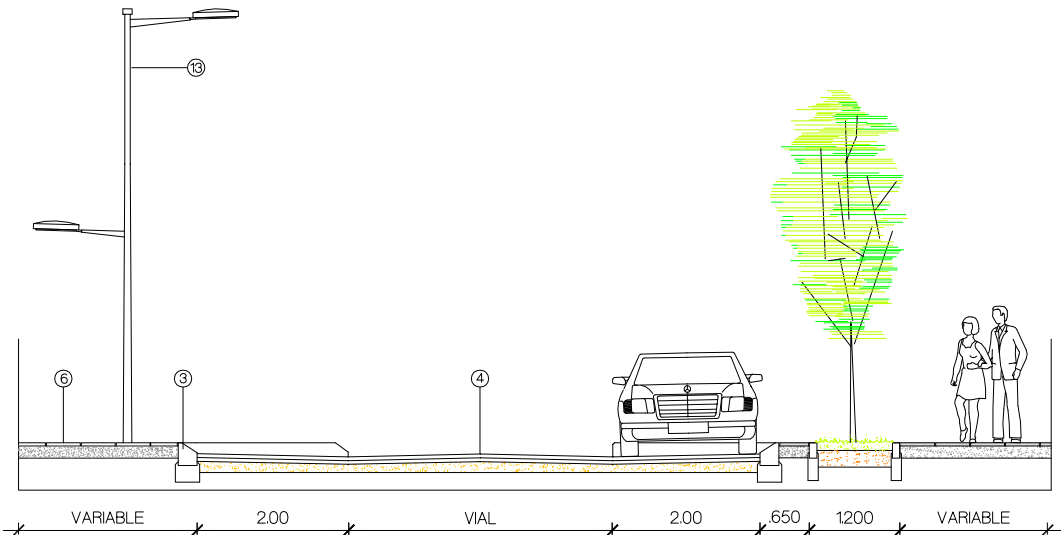
SECCIÓ PAS DE VIANANTS
