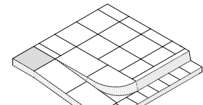
GUAL VIANANTS AXONOMÈTRICA PENDENT 12% SECCIÓ GUAL VIANANTS
