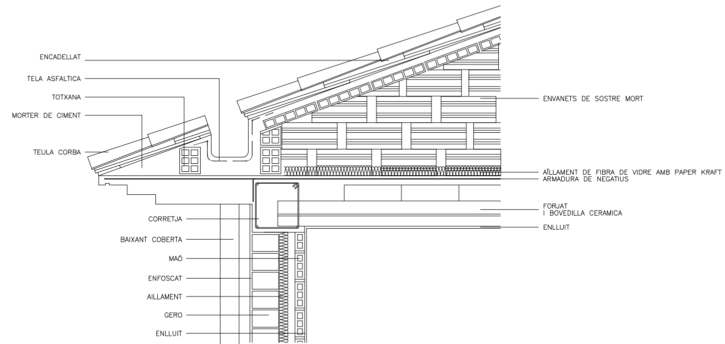
1 COBERTA INCLINADA AMB ALERO
