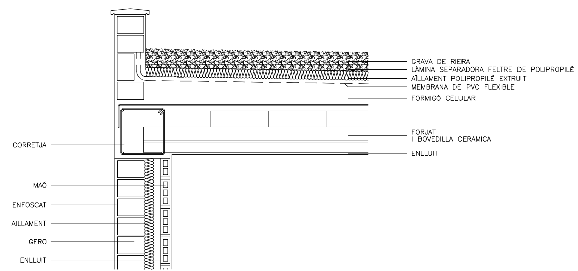
3 COBERTA INVERTIDA PLANA NO TRANSITABLE
