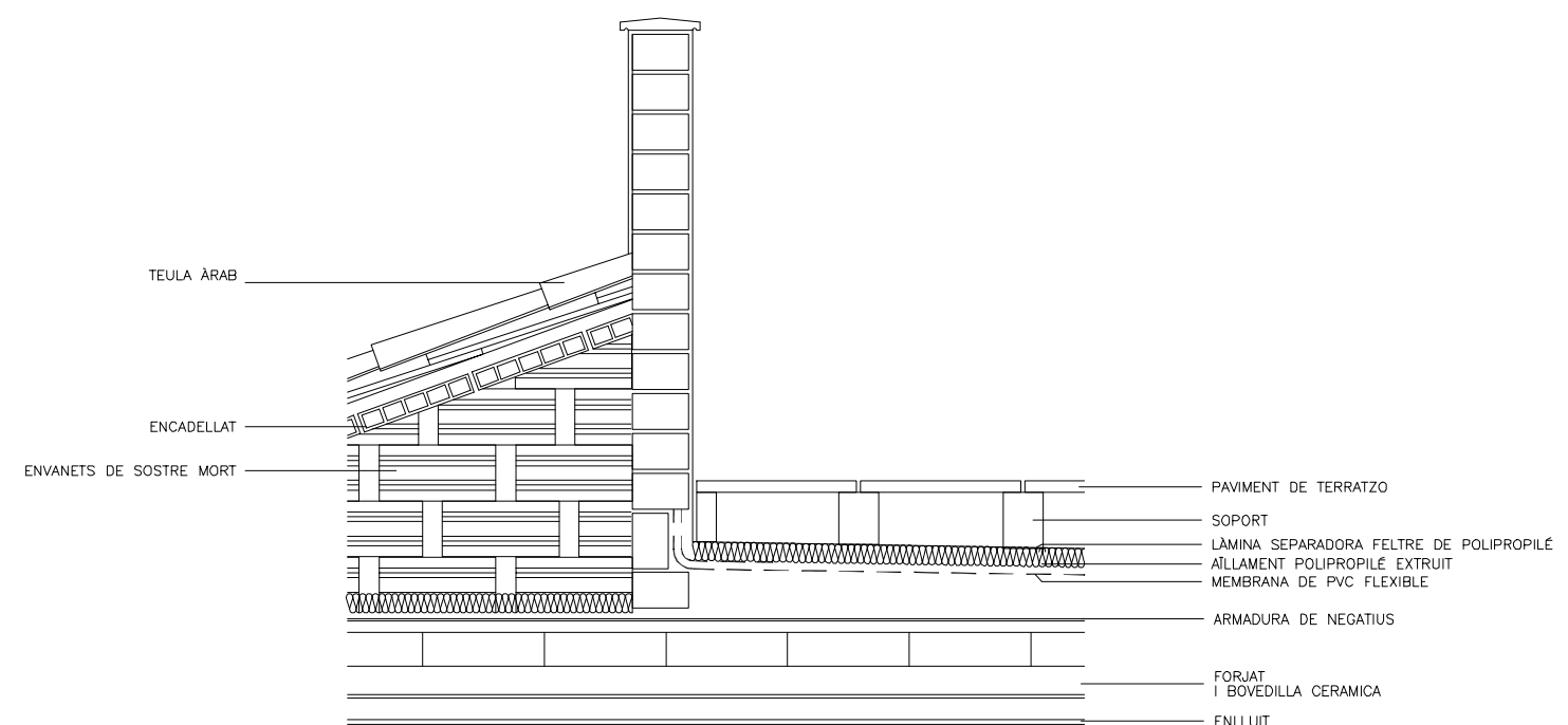
2 COBERTA INVERTIDA PLANA TRANSITABLE
