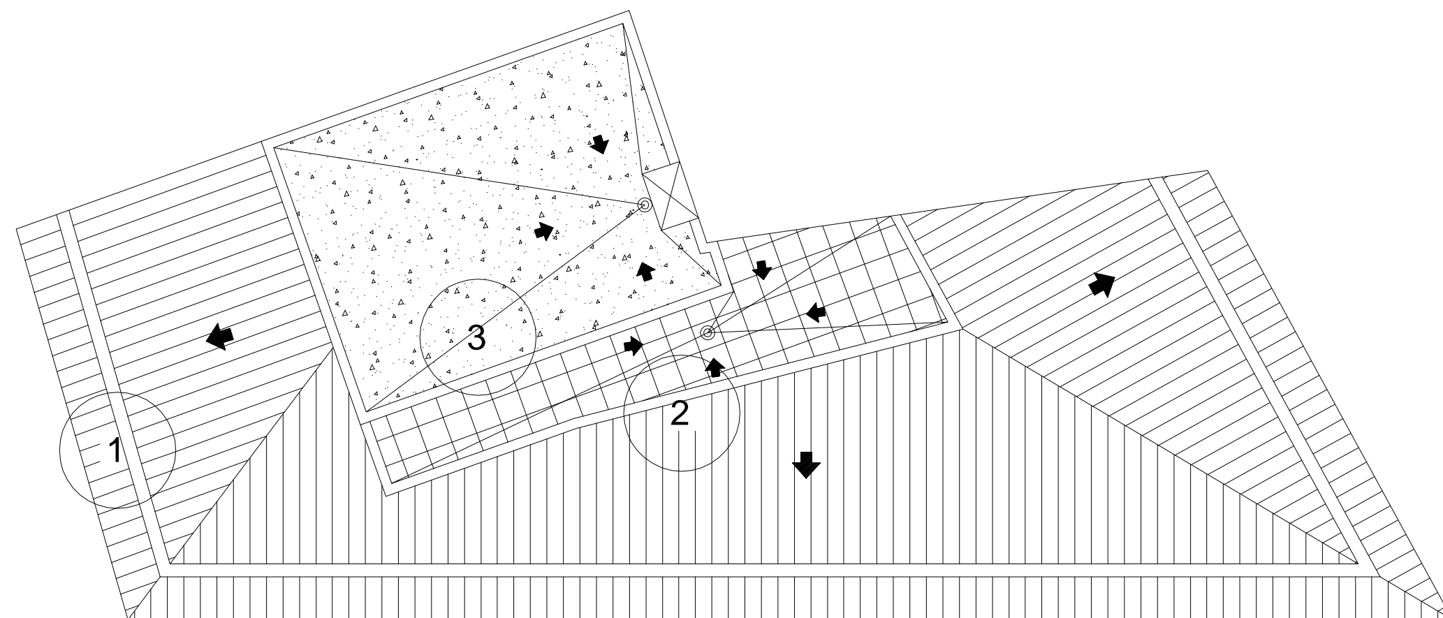
3 COBERTA INVERTIDA PLANA NO TRANSITABLE
