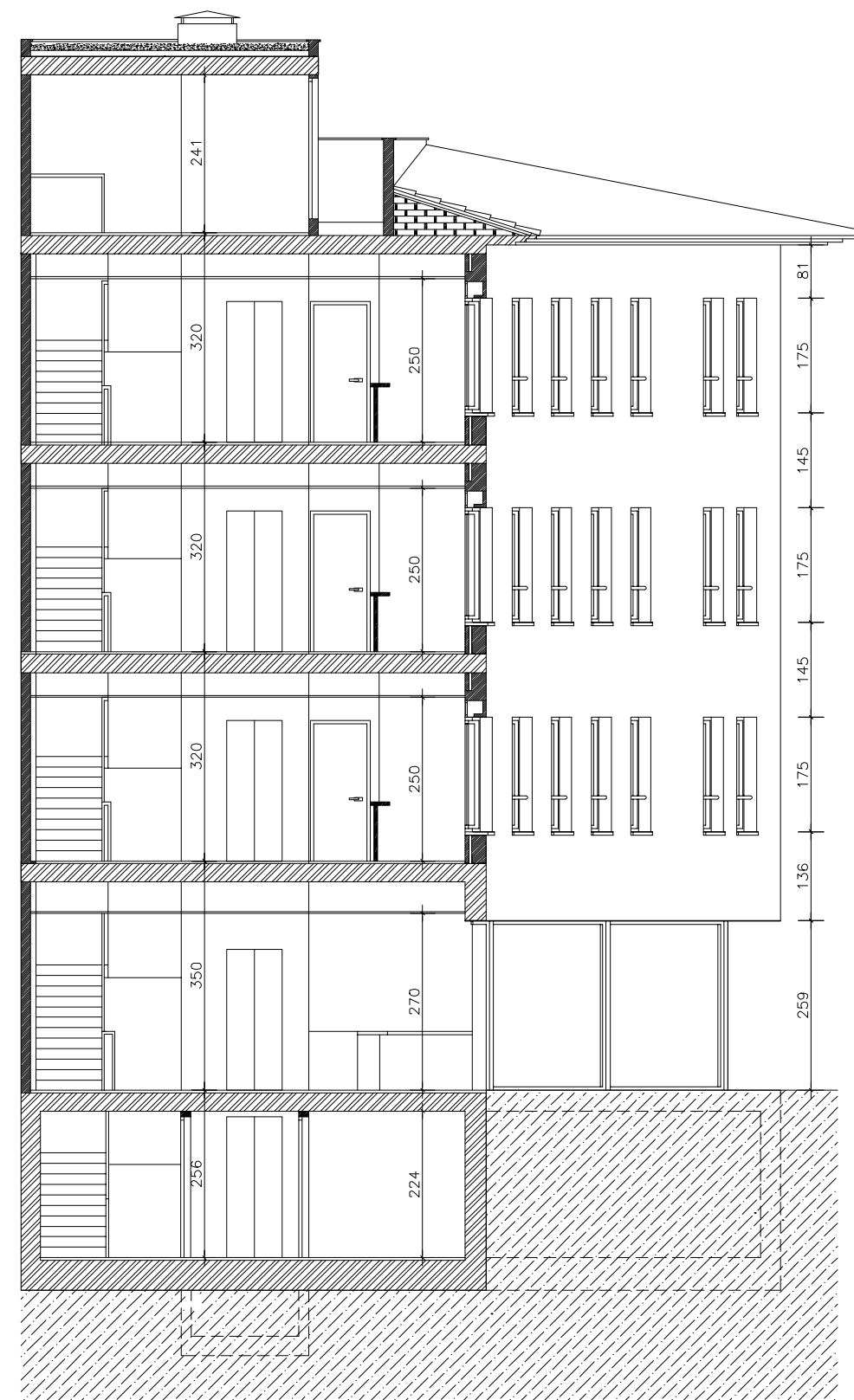
SECCIO A-A
